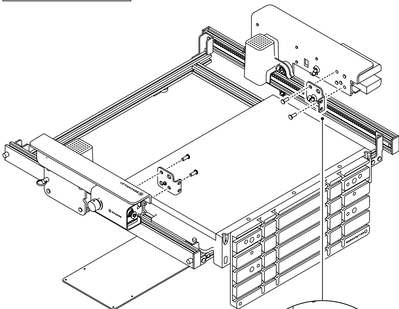
Skruv B (4x) Insexnyckel 4 mm
