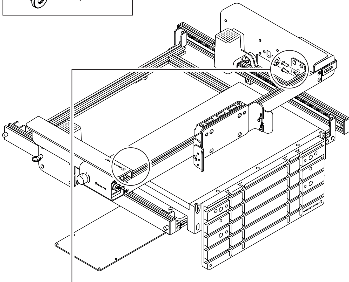
Skruv B (4x) Insexnyckel 4 mm
