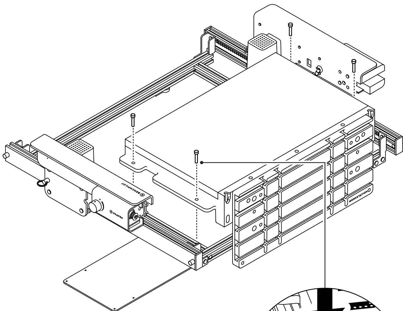
Skruv A (4x) Insexnyckel 4 mm
