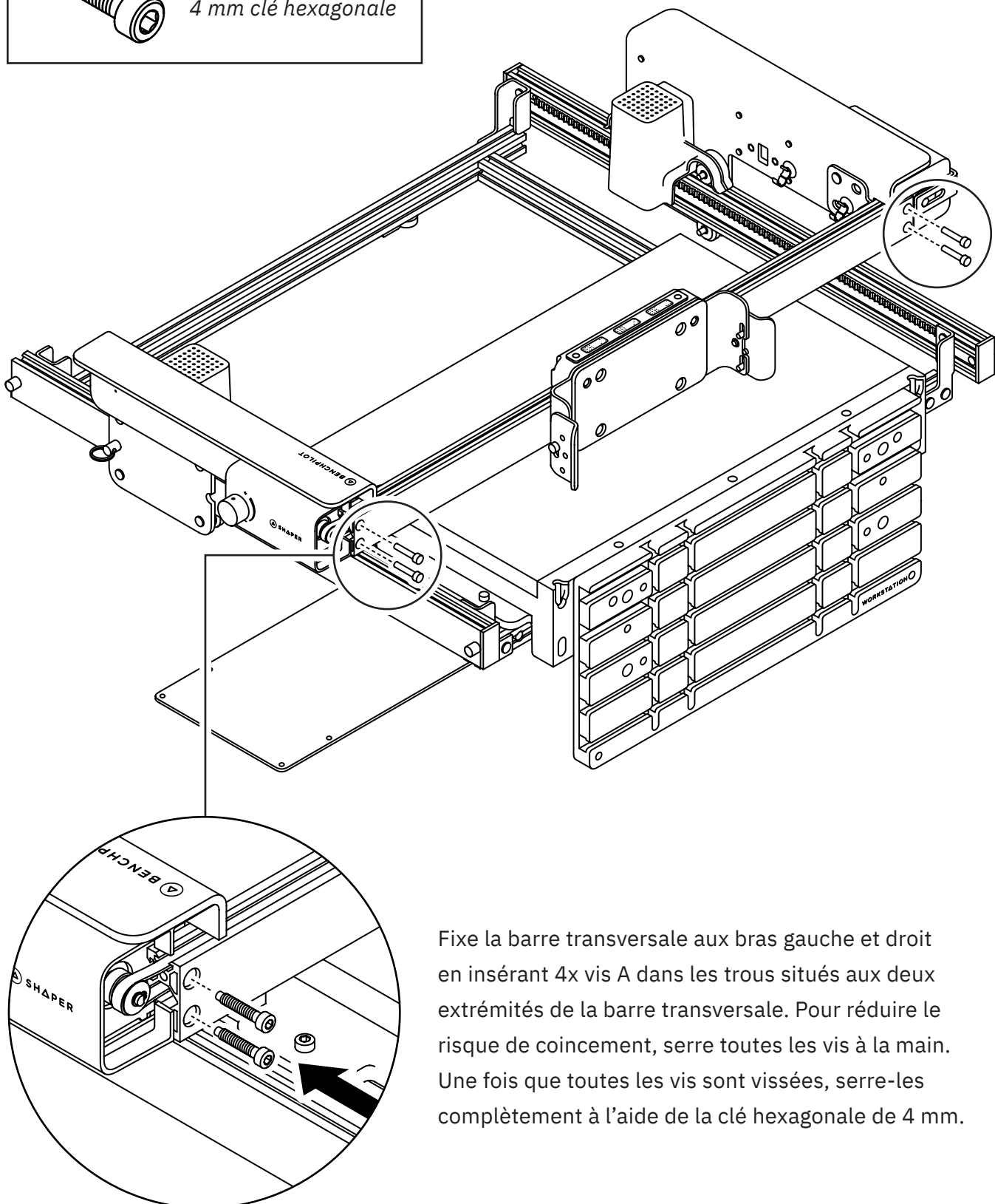
Vis A (4x) 4 mm clé hexagonale
